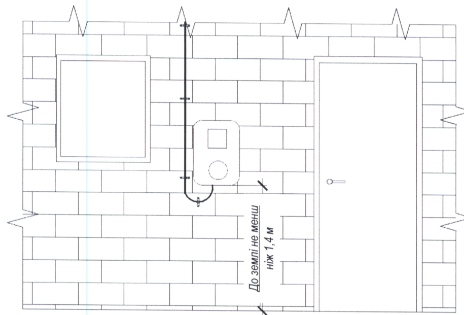
Розміщення ЗКОЕ на зовнішній стіні будівлі
