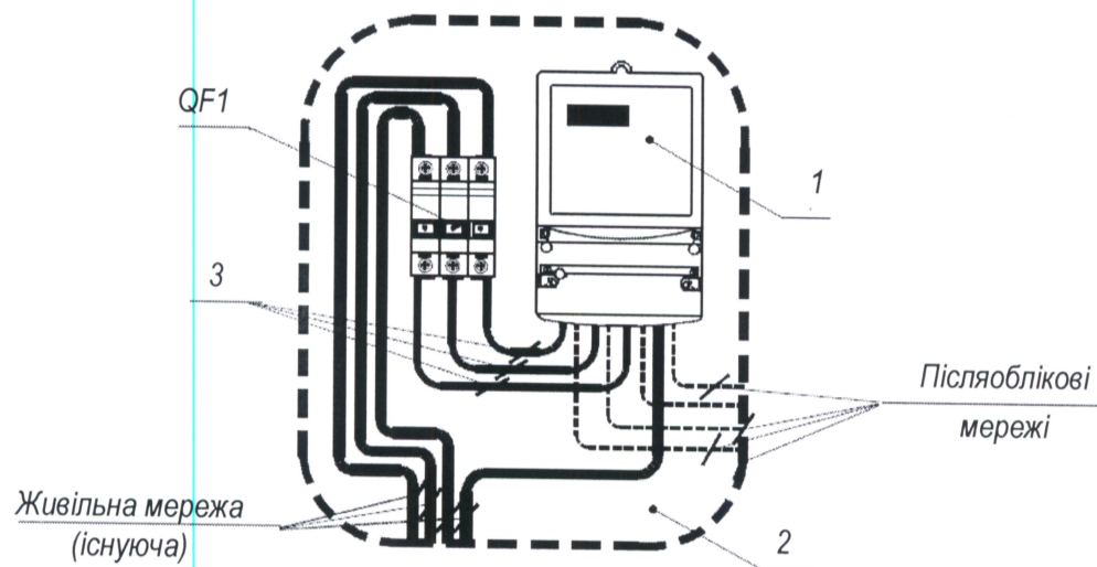
Монтажна схема ЗКОЕ
