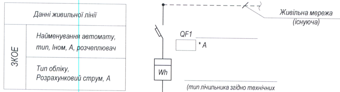
Принципова схема живильної мережі
